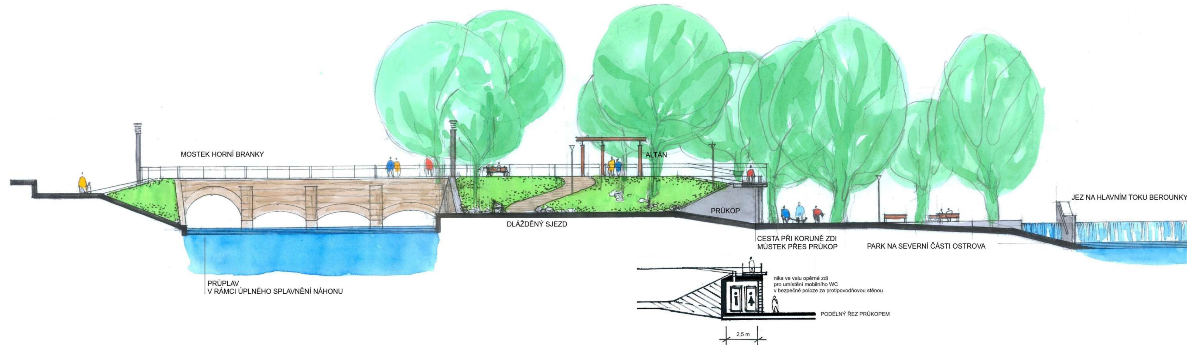
OSTROV PŘÍČNÝ REZ
